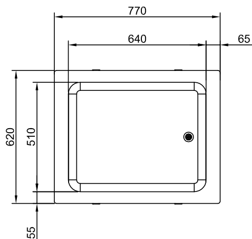
Boven aanzicht
